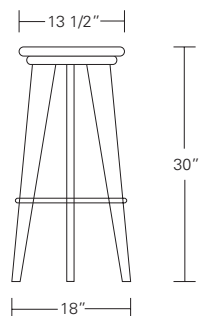
Top Stool
