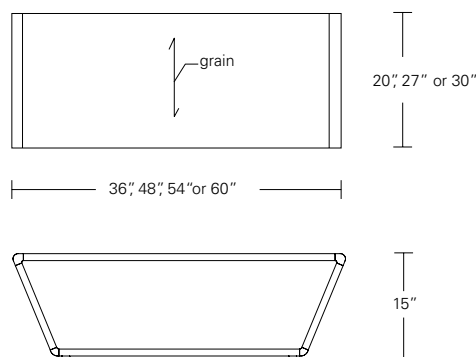
Contour Cocktail Table 36"W x 20"D x 15"H 48"W x 20"D x 15"H 54"W x 20"D x 15"H 48"W x 27"D x 15"H 54"W x 27"D x 15"H 60"W x 30"D x 15"H
