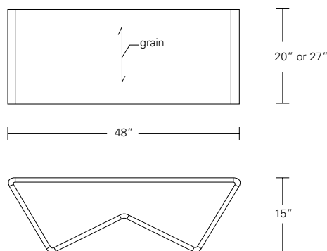
Zig Zag Table 48"W x 20"D x 15"H 48"W x 27"D x 15"H
